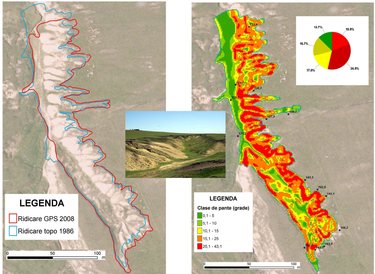
Fig. 7. Ravena Coada Găștii. Evoluția conturului ravenei în ultimii 22 ani (stânga). Distribuția geodeclivităților în aria ravenei (dreapta).
