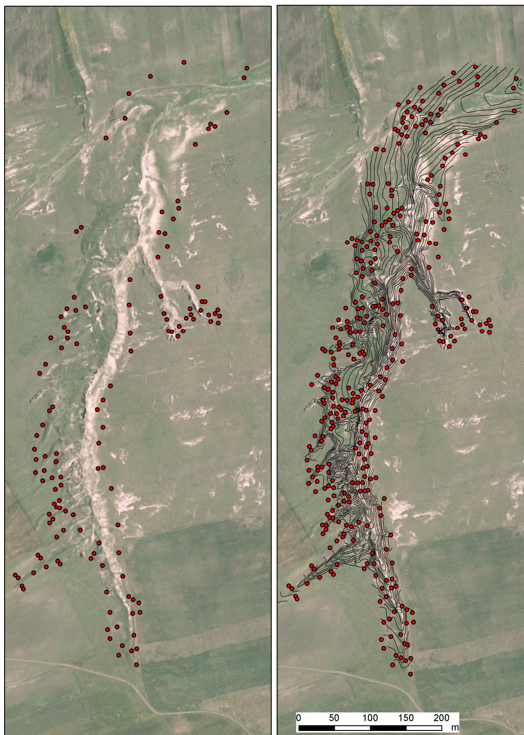
Fig. 8. Ravena Gurguiata Mare. Puncte folosite la interpolarea suprafeței inițiale (stânga); Puncte și curbe de nivel (echid. 1 m) folosite la realizarea modelului digital al ravenei (dreapta).
