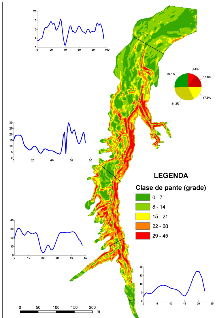
Fig. 6. Harta geodeclivității în aria Ravenei Gurguiata Mare.
